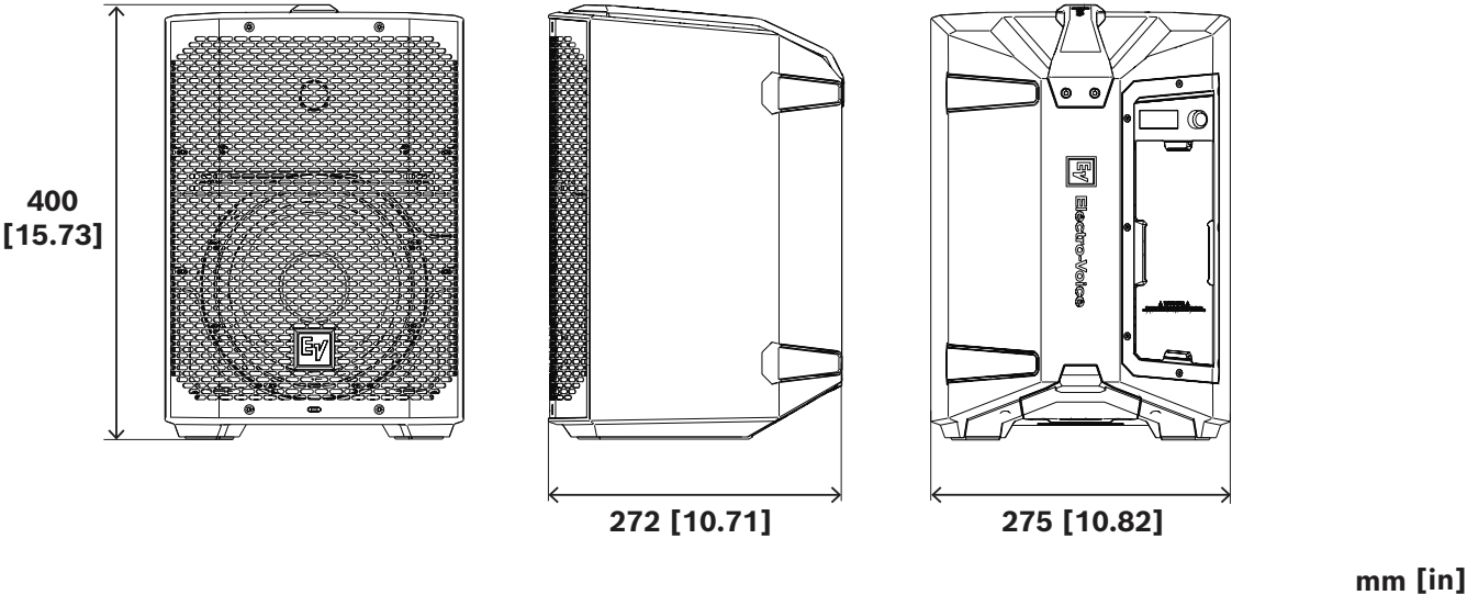
Fig. 1: Dimensions
