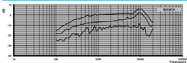
Hình 1: Hồi đáp tần số (Góc mở: 0, 90 và 180 độ)
