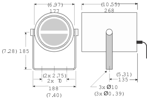
Kích thước tính theo mm (in)
