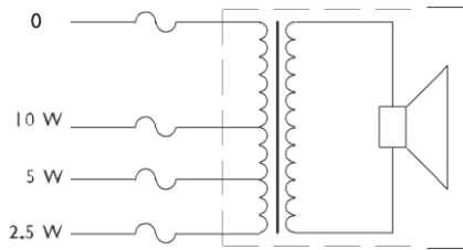
Sơ đồ nối mạch
