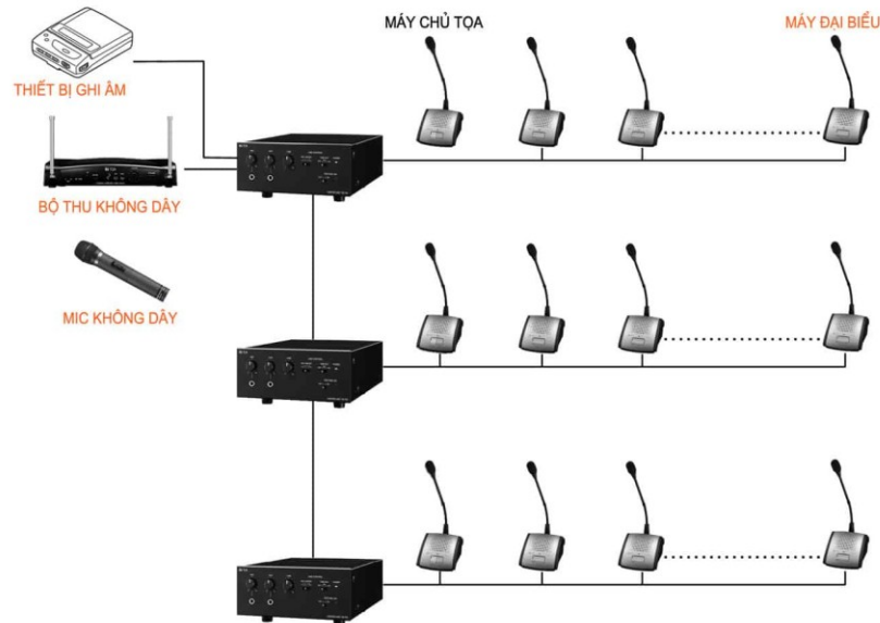
Sơ đồ âm thanh hội thảo cơ bản
